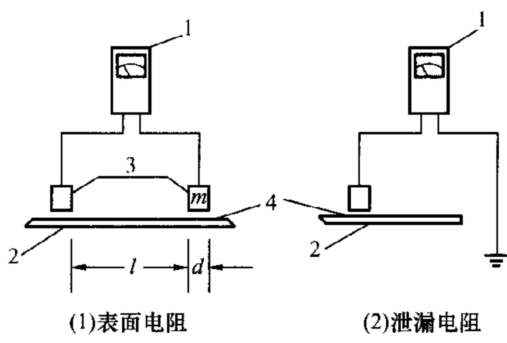
图 E. 9. 3 表面导静电性能测试装置
